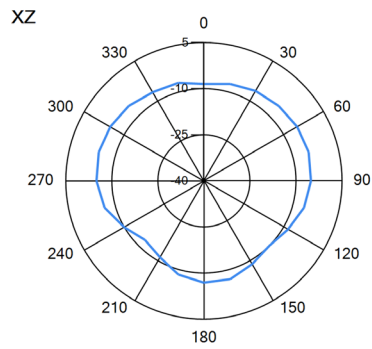
— 433MHz
